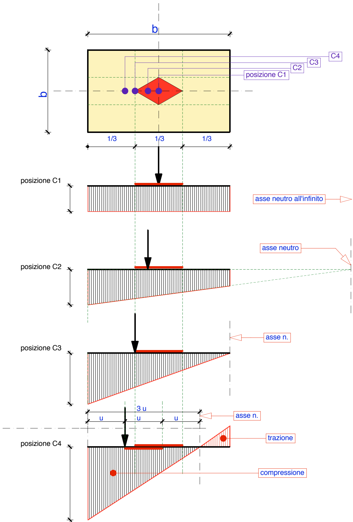
DIAGRAMMI DELLE SOLLECITAZIONI IN UNA SEZIONE RETTANGOLARE AL VARIARE DELLE LINEE DI AZIONE DEL CARICO "P" ENTRO E FUORI IL NOCCIOLO CENTRALE DI INERZIA
